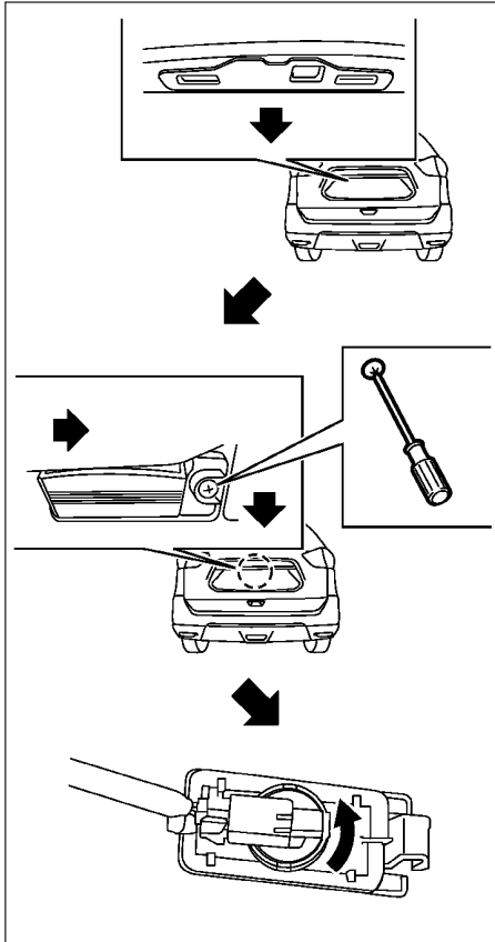
چراغ پلاک
