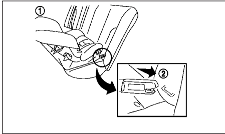
گام‌های ۱ و ۲
