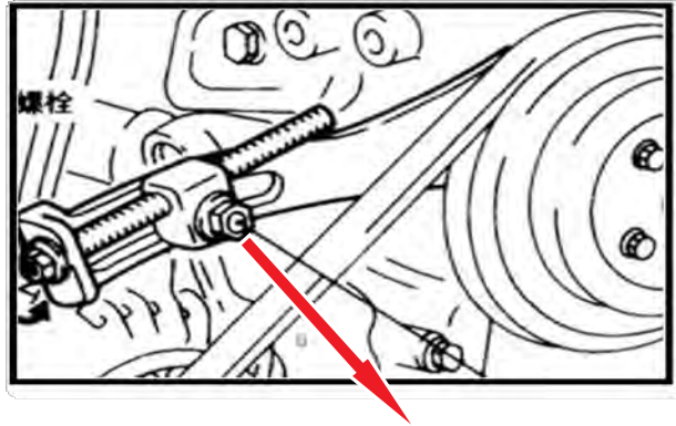
پیچ تنظیم تسمه دینام
