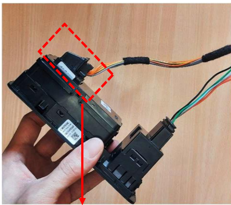
مجموعه کانکتور و سوئیچ پدل
