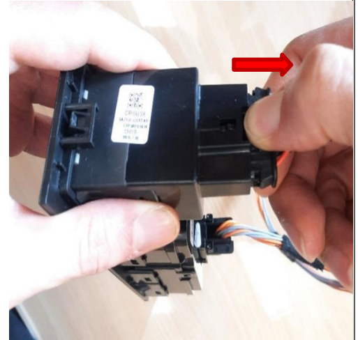
مرحله کشیدن کانکتور
