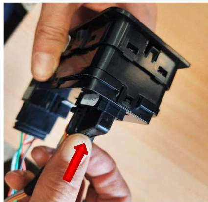
مرحله فشردن قفل کانکتور
